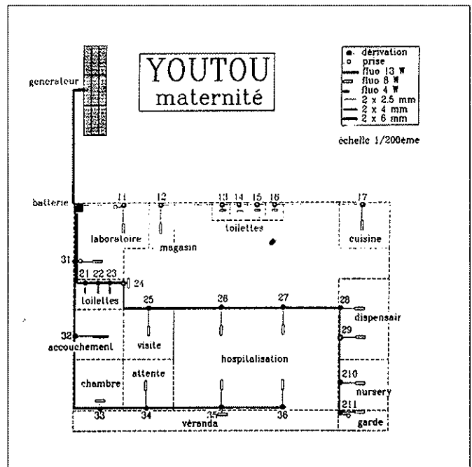
Plan de la maternité de Youtou connectée à son générateur.
